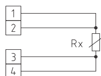
1x Vierleiterschaltung
